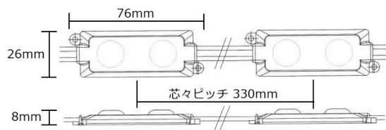
外形寸法
