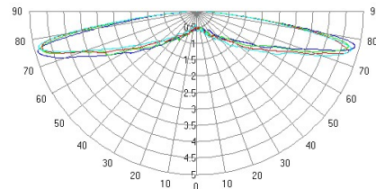
配光図
